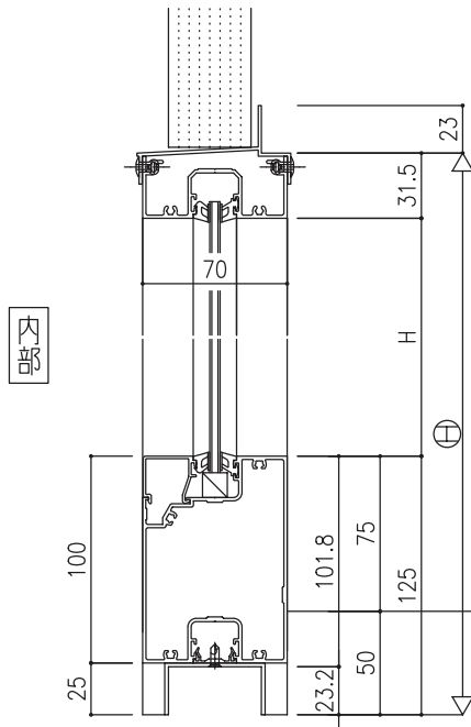
土台パネル納まり
