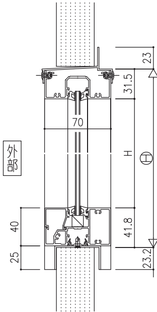
パネル納まり
