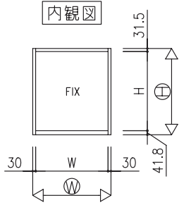
パネル納まり
