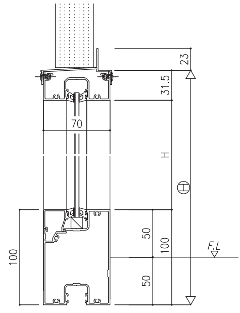
巾木納まり
